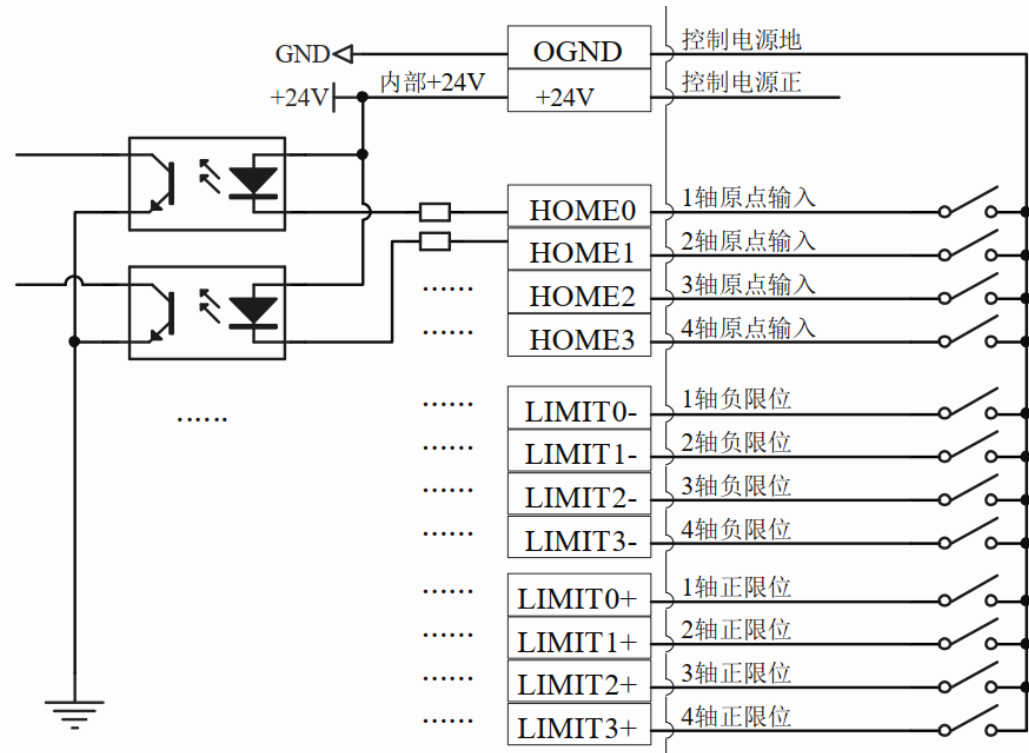
图 3.5.1 数字输入输出配线示意图
