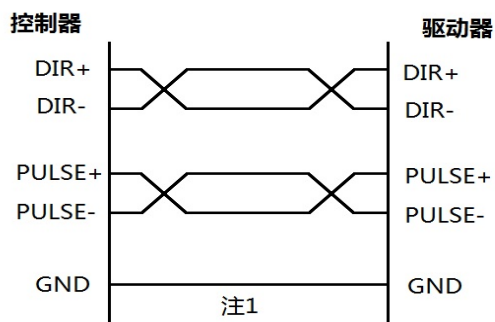
图 3.2.3 脉冲输出差分接法示意图
